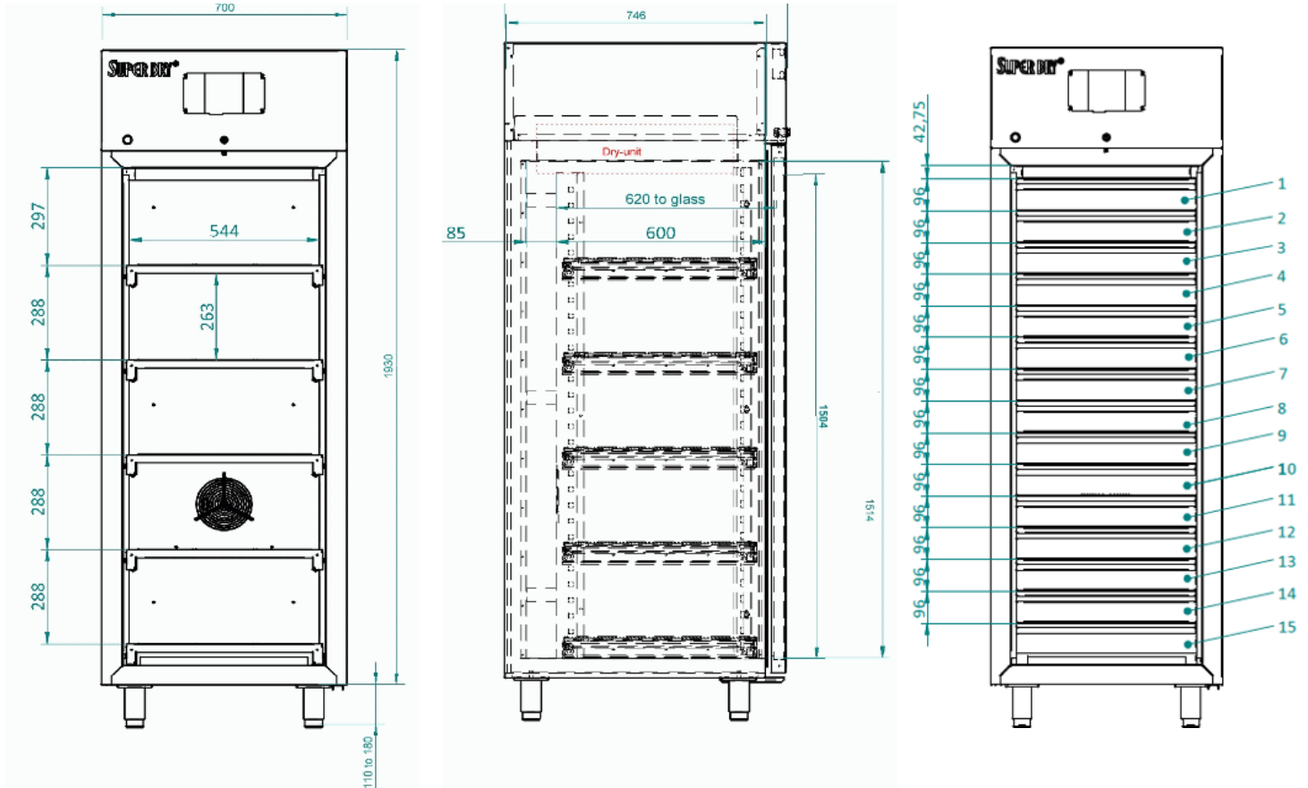
Frontansicht
